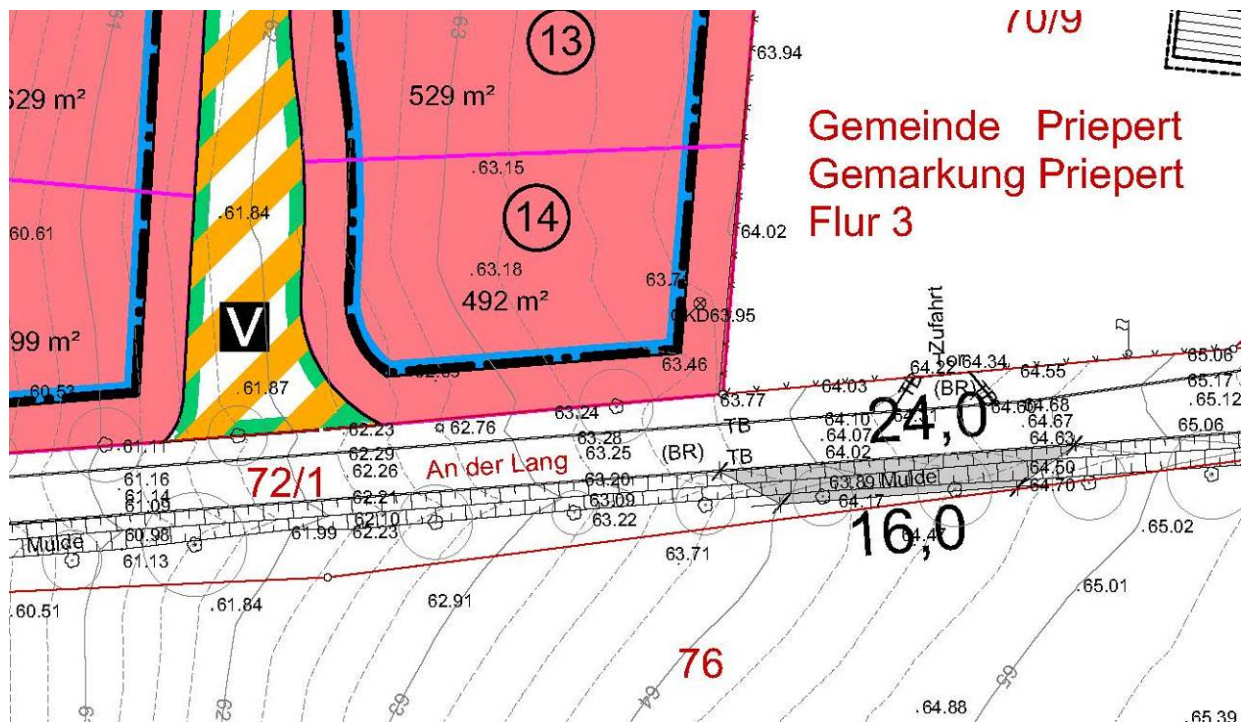
Abb. 15: Geplante Einmündung der Erschließungsstraße in die Straße „An der Lang“ und geplante Ausweichstelle an der Straße „An der Lang“
